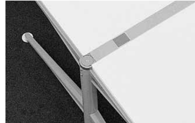
Canalizzazione coplanare al piano (gamba doppia). Coplanar channel to the top (double leg). Canalisation coplanaire au plateau (pied double).
